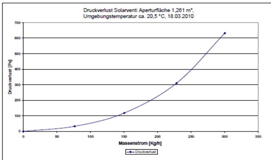
Abbildung 17: Druckverlustkennlinie aufgetragen über Massenstrom in kg/h
