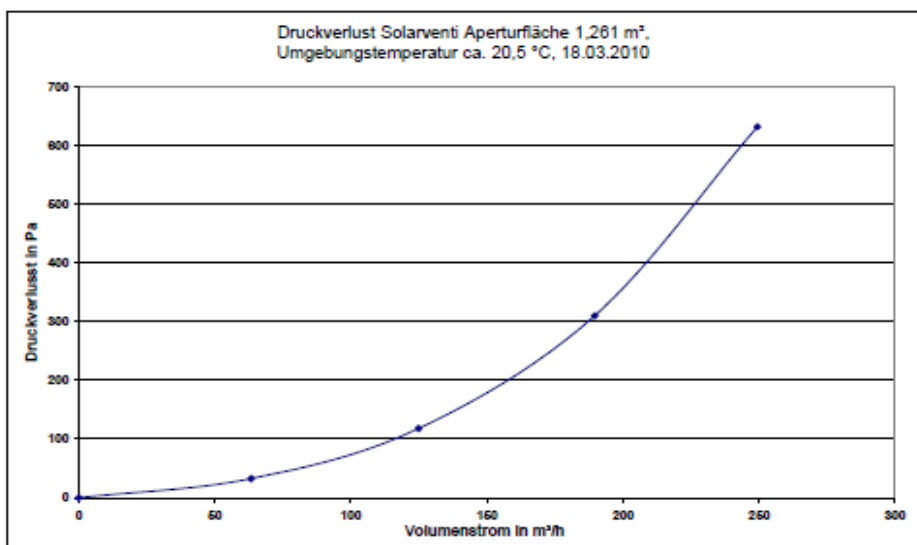
Abbildung 16: Druckverlustkennlinie aufgetragen über Volumenstrom in m 3 /h
